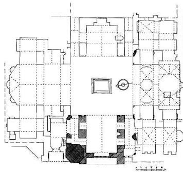
نقشه ۲. مسجد جامع گز - بخش هاشور خورده از سلجوقی (ویلبیر، ۱۳۶۵: شکل ۲۹)
