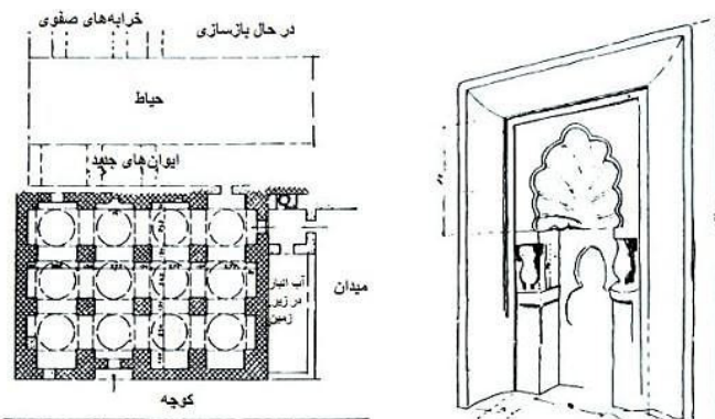
طرح ۱. محراب مسجد صدراسلامی شاپورآباد (سیرو، ۱۳۵۷: ۳۶۹) نقشه ۴. بنای اولیه مسجد شاپورآباد (سیرو، ۱۳۵۷: ۳۶۹)
